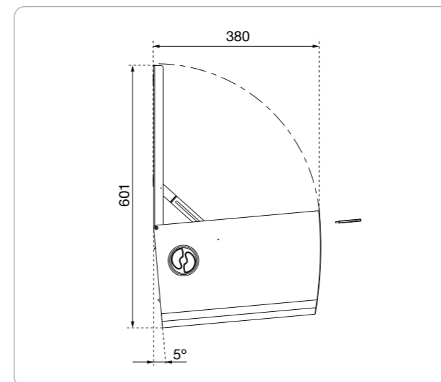
Technische Zeichnung.
